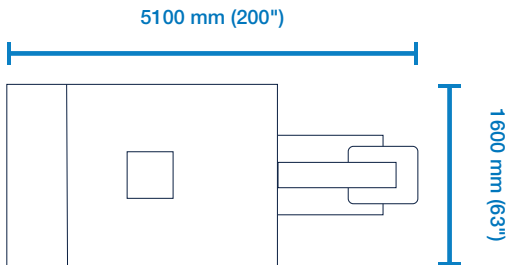
Draufsicht
