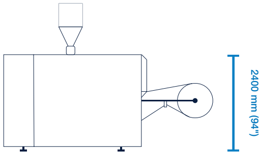
Seitenansicht
